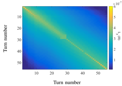
Fig. 7. Inductance matrix.
