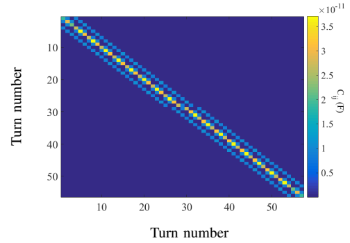
Fig. 6. capacitance matrix.
